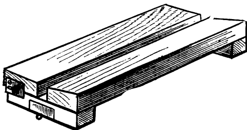
Рис. 40. Универсальная расправилка.
