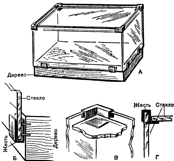
Рис. 76. Изготовление разборного стеклянного колпака:
