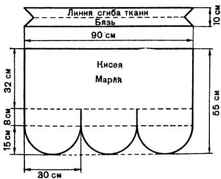
Рис. 3. Выкройка мешка энтомологического сачка.
