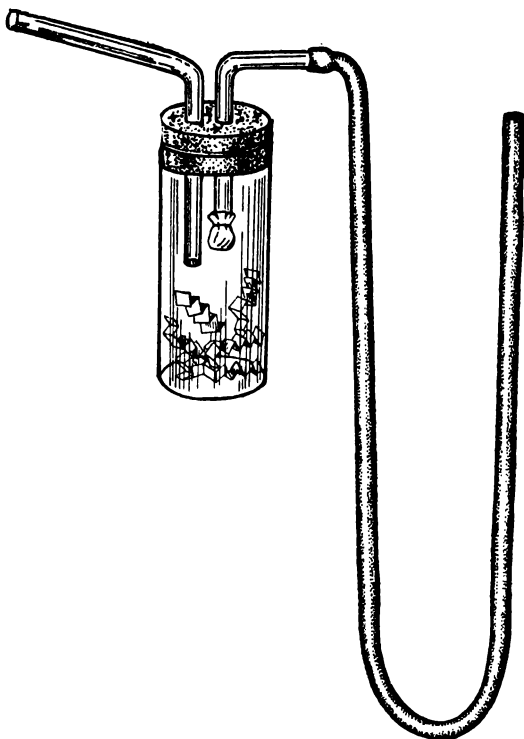
Рис. 9. Эксгаустер.
