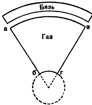
Рис. 59. Выкройка планктонной сети.
