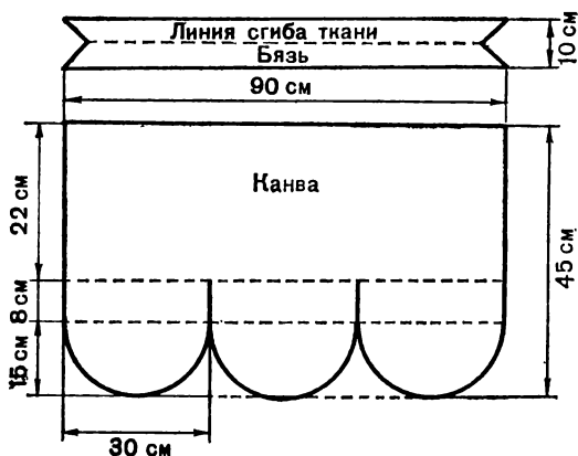
Рис. 53. Выкройка мешка водного сачка.
