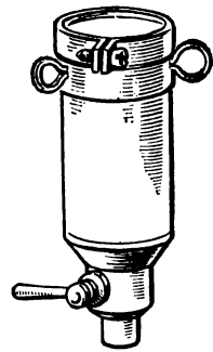
Рис. 60. Металлический стакан для планктонной сети.
