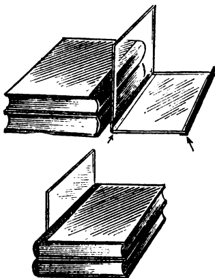
Рис. 74. Соединение стенок полосками материи при изготовлении стеклянного колпака.
